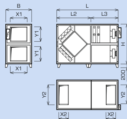
PARAPETNÍ (pohled z čela) Basic 12 100 až 15 100 provedení 12/x a 13/x
