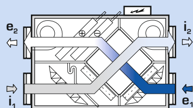
větrání s rekuperací s dohřevem (s chlazením)
