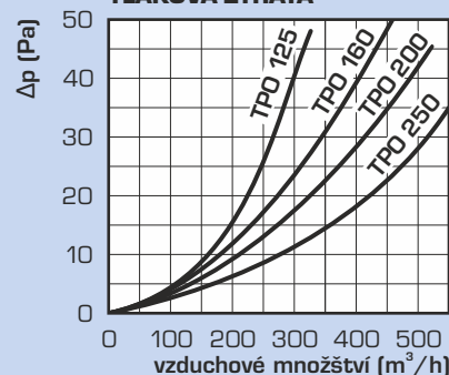
TLAKOVÁ ZTRÁTA
